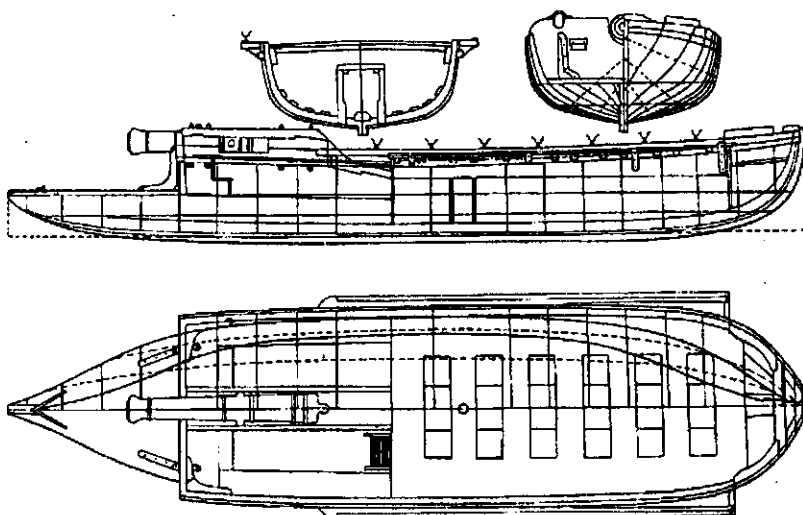
Трофейный шведский кононерский иол
