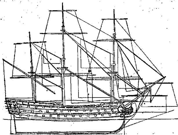
Корпус и боковой вид 100-пушечного корабля «Пётр I и II» с рангоутом (чертеж утвержден Петром Михайловым)
