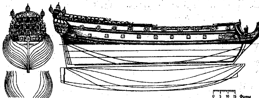
Корабль «Страфорд»
