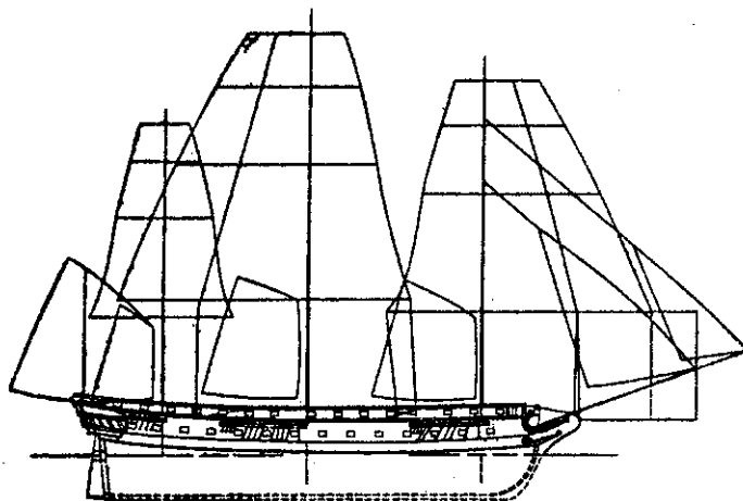
Фрегат «Штандарт»
