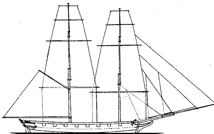
Яхта «Нева»
