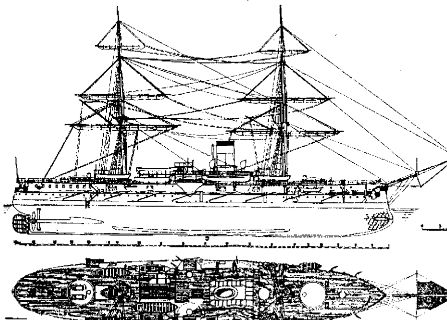
Броненосный фрегат «Адмирал Нахимов»
