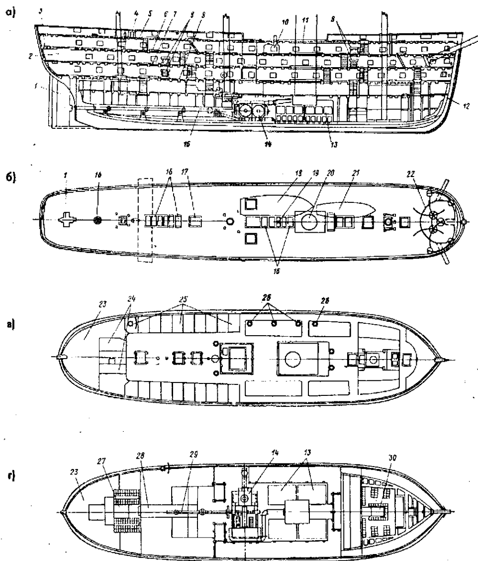
Чертежи общего расположения 1 1 1-пушечного парусно-винтового корабля
