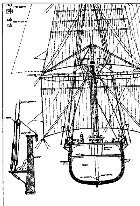
Шлюп «Мирный». Разрез по носу
