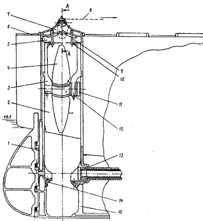
Устройство для подъема гребного винта на фрегате «Герцог Эдинбургский»
