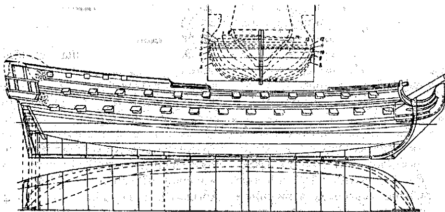
Чертеж корабля постройки 1709 г.
