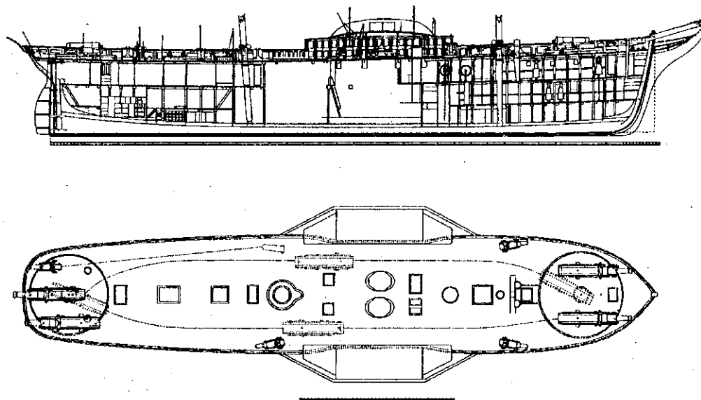
Пароходо-фрегат «Громоносец»
