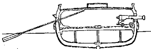
Разрез прама «Олифант» (рис. А.Е. Лютова)
