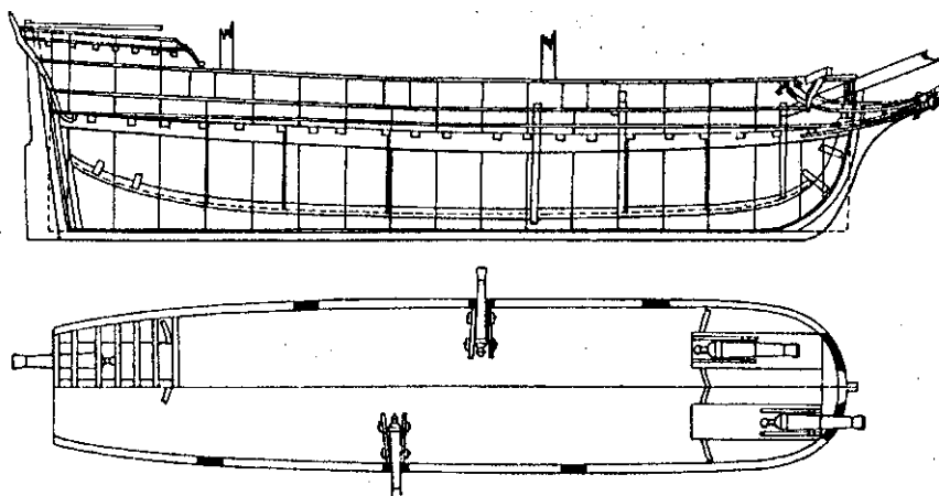
Русская полушебека
