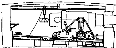
11-дм пушка Круппа обр. 1867 г. в башенной установке для башенных фрегатов типа «Адмирал Грейг»
