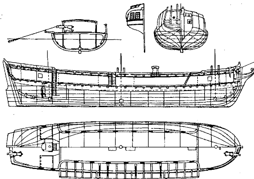
«Секретные» суда «Охранительное» и «Наступательное»
