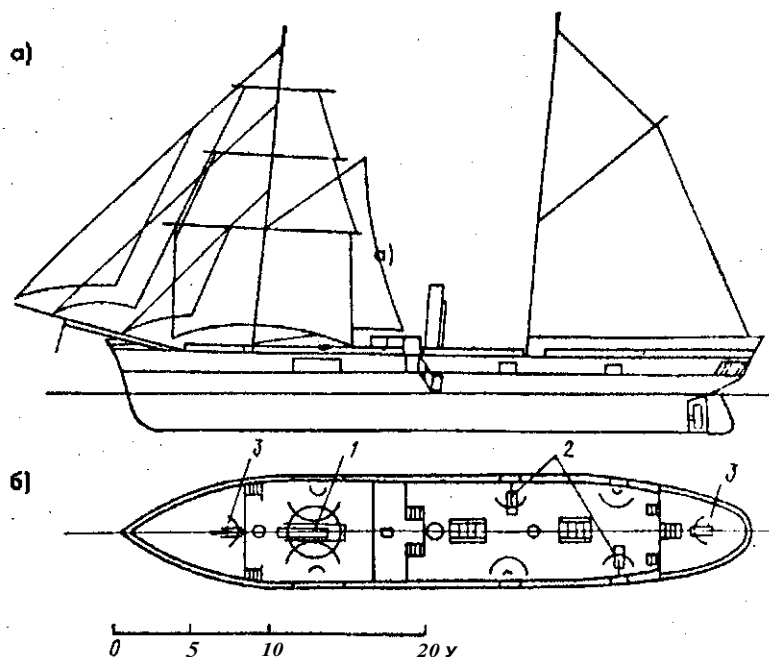
Винтовая канонерская лодка «Нерпа»: а — вид с боку и парусное вооружение; б — план верхней палубы. 1 — 6-дм орудие; 2 — 9-фн орудия; 3 — 4-фн орудия
