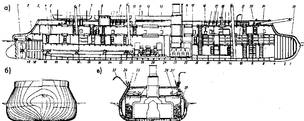
Броненосная батарея «Первенец»:
