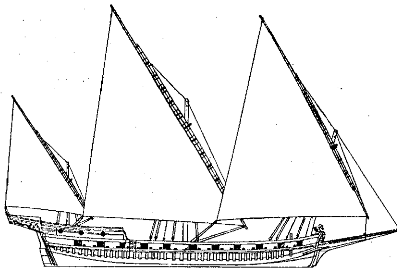
Русская шебека «большого типа» (рис. А.Е. Лютова)
