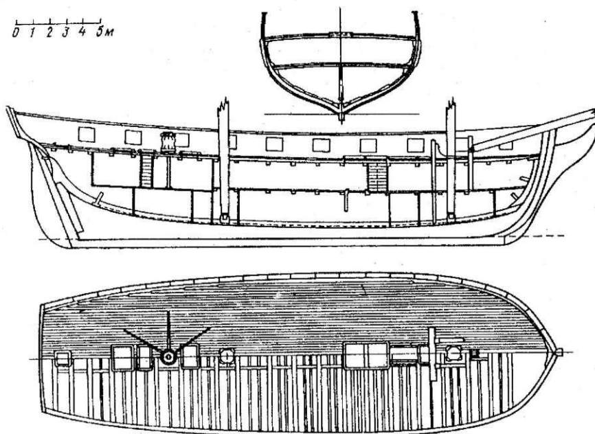
Мидель-шпангоут, продольный разрез и вид сверху брига «Феникс»
