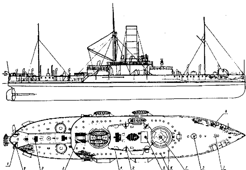
Монитор «Пётр Великий» после ремонта в Англии в 1882 г.:
