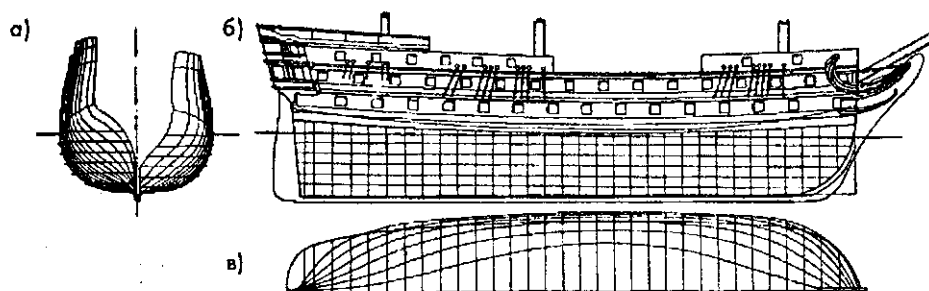
Чертеж 74-пушечного корабля «Александр Невский»:
