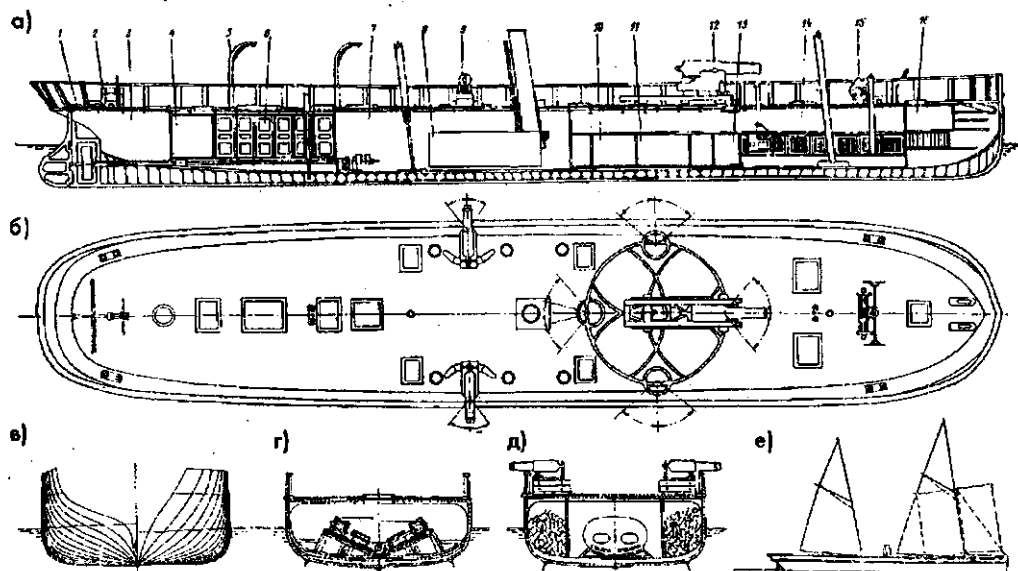
Канонерские лодки «Секира» и «Пищаль»;
