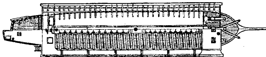
План палубы галеры «Двина»
