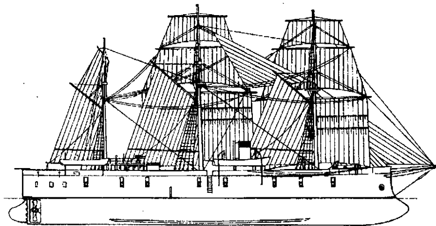
Броненосная плавбатарея «Кремль»
