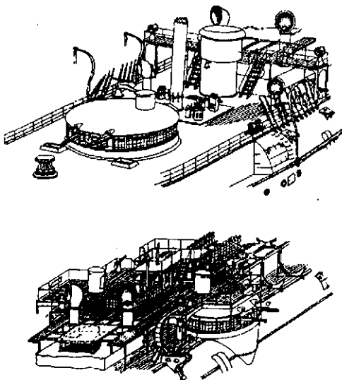
203/35-мм (8-дм) пушка в барбетной установке фрегата «Адмирал Нахимов»
