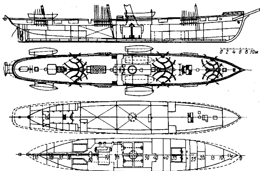
Клипер «Стрелок» (1879 г.)
