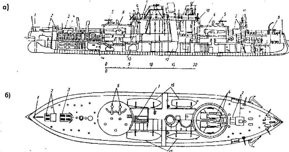
Двухбашенная лодка «Чародейка»:
