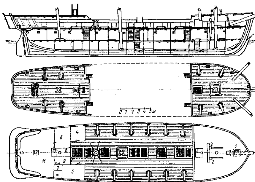
24-пушечный фрегат «Надежда»
