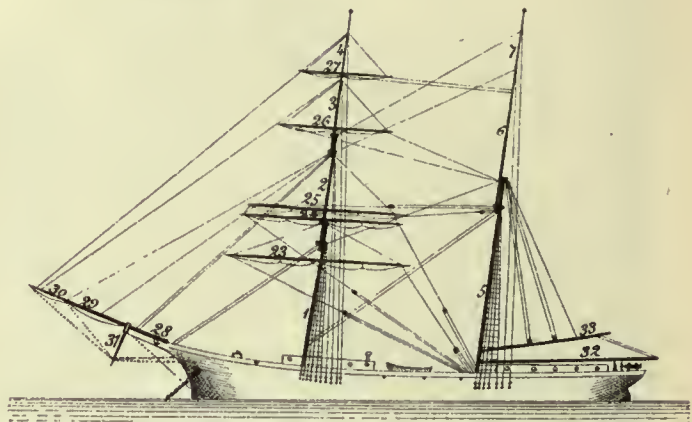
Fig. 132. Barkentine Spars
