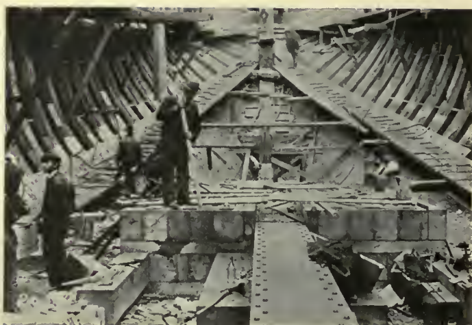
Fig. 84. Steel Keelson
