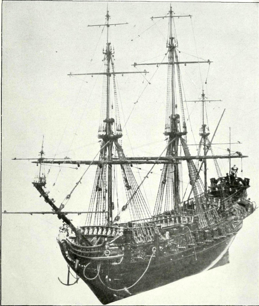
Abb. 28. Kurbrandenburgische Fregatte „Friedrich Wilhelm zu Pferde“ 17. Jahrh. n. Chr.
