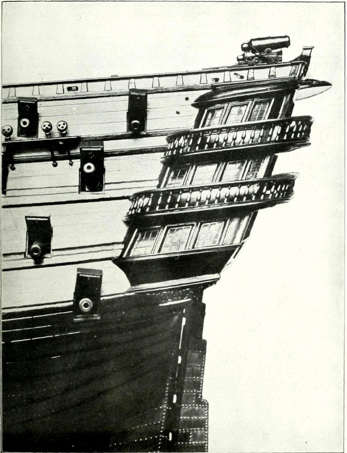
Abb. 34. Heckansicht zu Abb. 32
