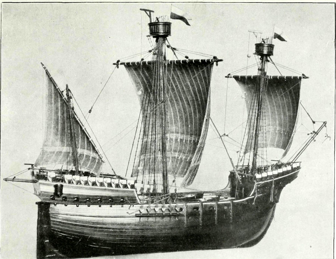
Abb. 24. Lübecker Hansa-Kogge 13.—15. Jahrh. n. Chr.
