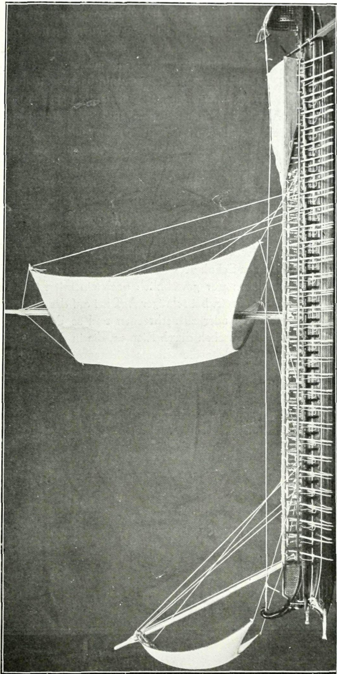
Abb. 9. Attische Triere 5.-4. Jahrh. v. Chr.
