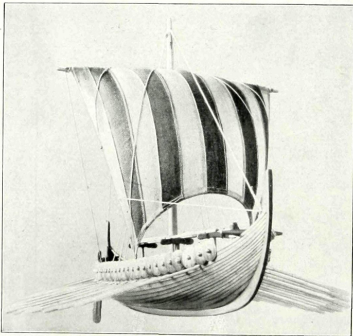
Abb. 22. Luvansicht zu Abb. 20
