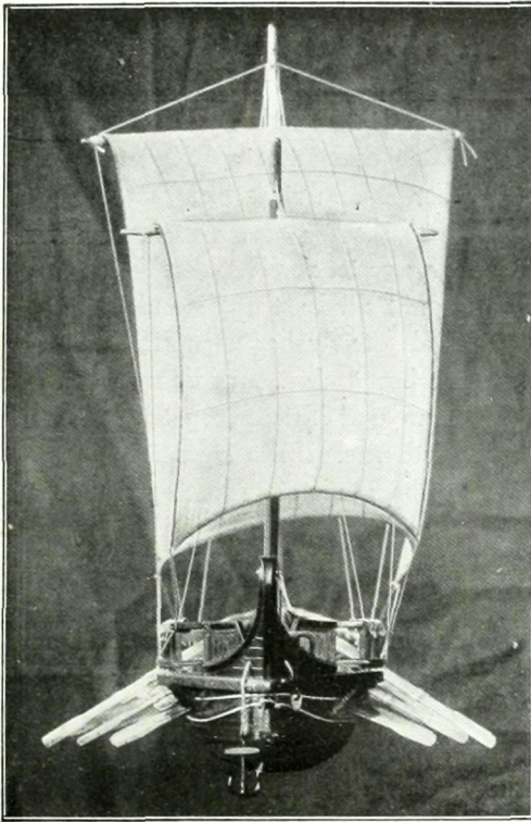
Abb. 14 u. 15. Vorder- und Achteransicht zu Abb. 9
