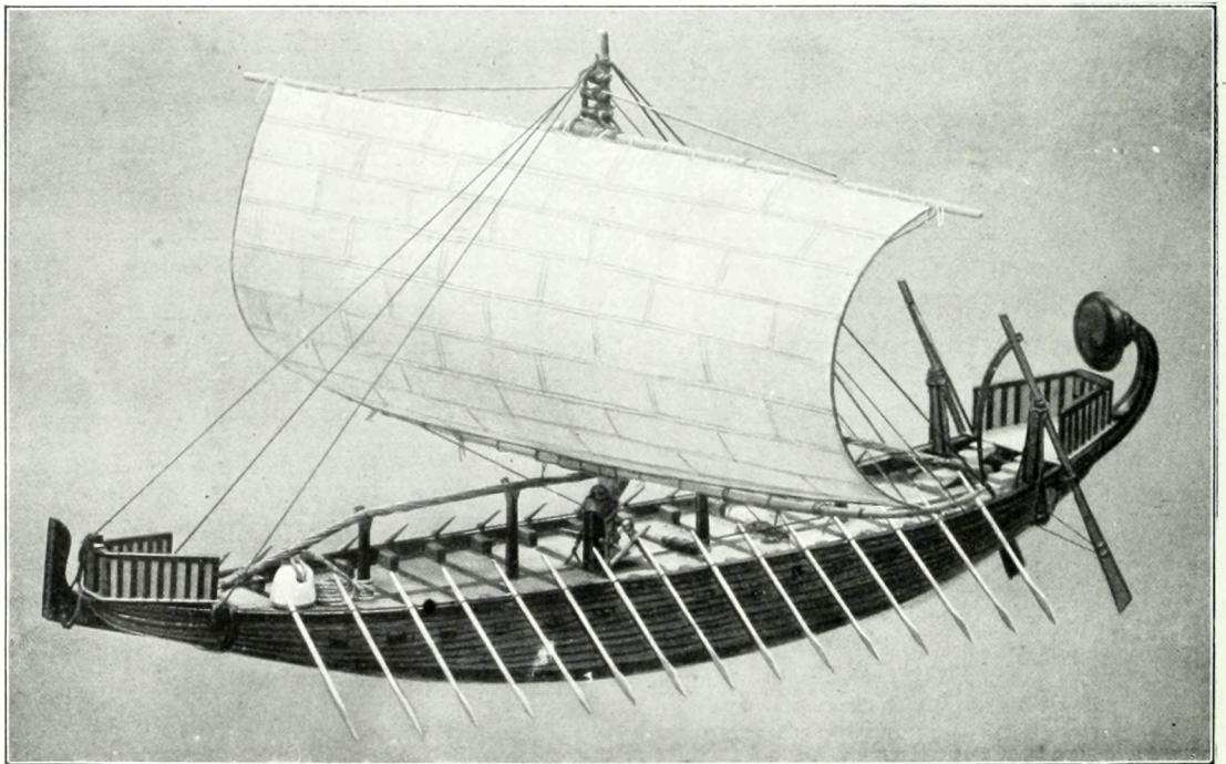
Abb. 5. Leeansicht zu Abb. 6
