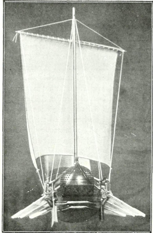
Abb. 14 u. 15. Vorder- und Achteransicht zu Abb. 9
