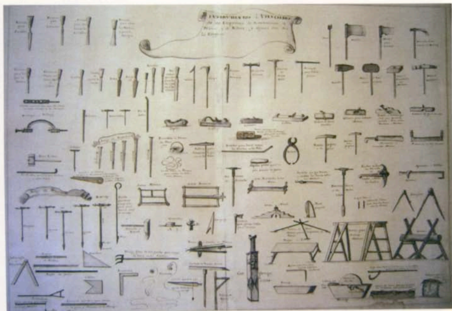
Instrumentos y utensilios de los carpinteros de construcción y ribera. Álbum del Marqués de la Victoria, AP.
