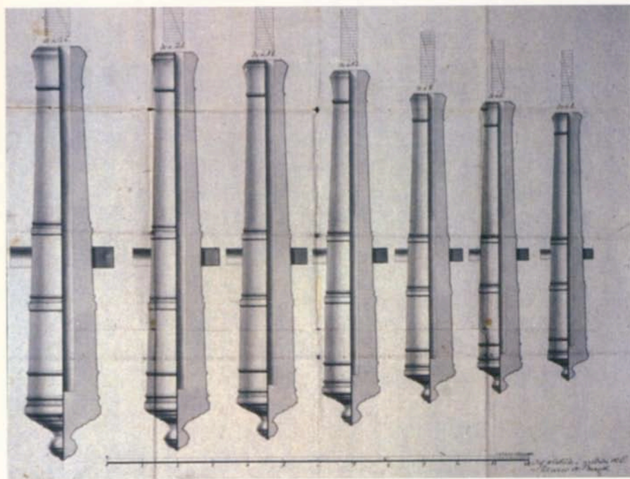
Dimensiones de distintos cañones de hierro colado para el servicio de la marina, 1752. Dibujo cedido amablemente por José Maza Uslé y Luis Villoslada
