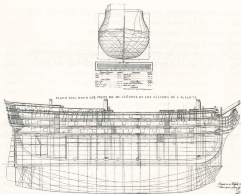
Navío de 112 cañones de últimos del siglo XVIII. A.P.
