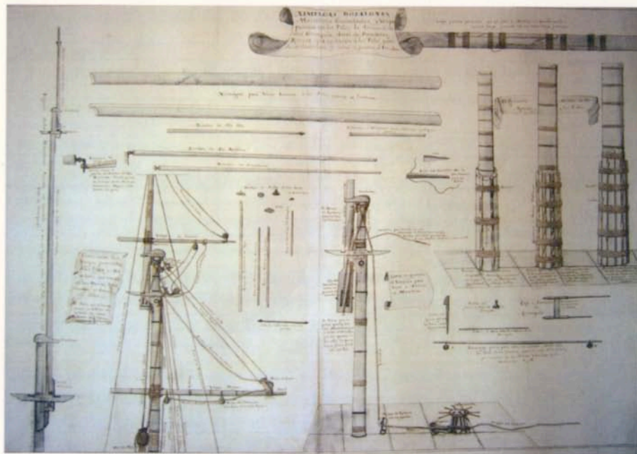
Representación y figura de las gimelgas, botalones de alas y rastreras y de desatracar, astas de banderas, etc. Álbum del Marqués de la Victoria, AP.
