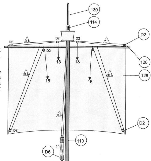
Mainmast / Гротмачта
