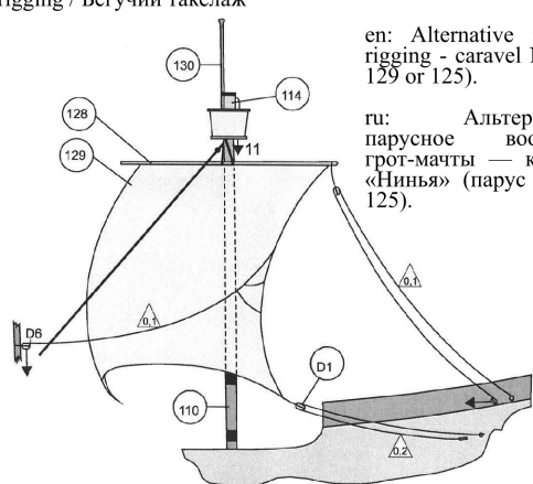
Running rigging / Бегучий такелаж
