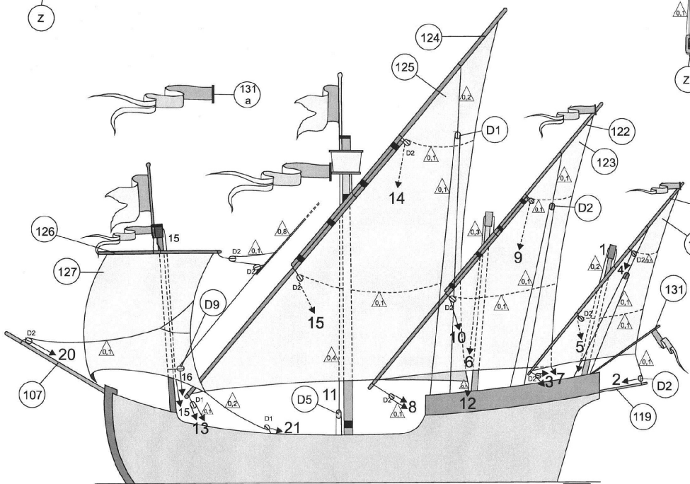
Running rigging / Бегучий такелаж
