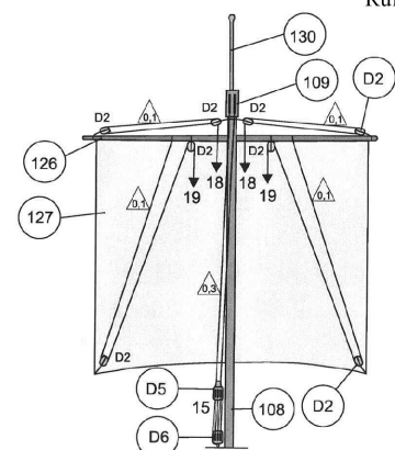
Foremast / Фокмачта
